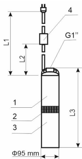
Obr.1 Rozměry a připojovací rozměry 1 – čerpací díl, 2 – filter, 3 – elektrický motor, 4 – kondenzátorni box.
