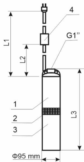
Obr.1 Rozměry a připojovací rozměry 1 – čerpací díl, 2 – filter, 3 – elektrický motor, 4 – kondenzatorní box.
